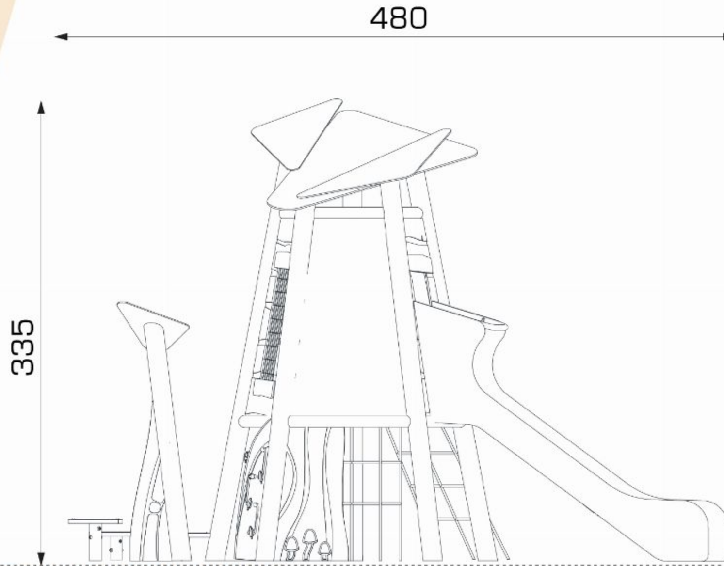
ÖN GÖRÜNÜŞ / FRONT VIEW
