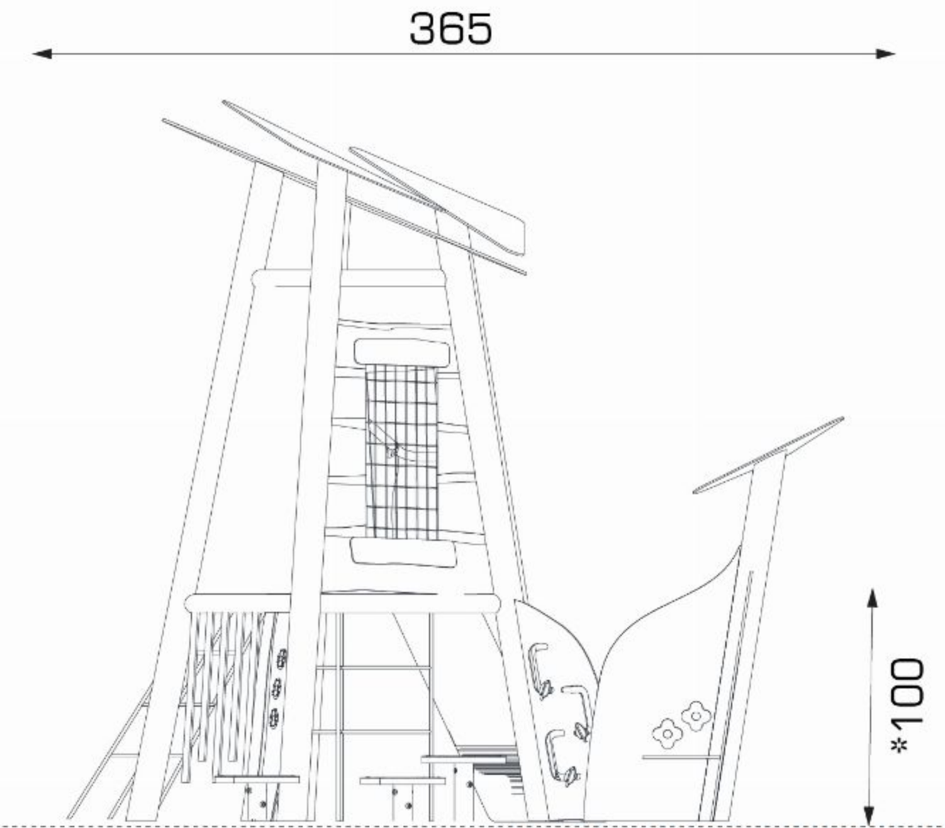
YAN GÖRÜNÜŞ / SIDE VIEW
